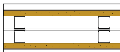
Metallkonstruktion Doppelständerwand
