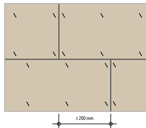
Plattenstoß
