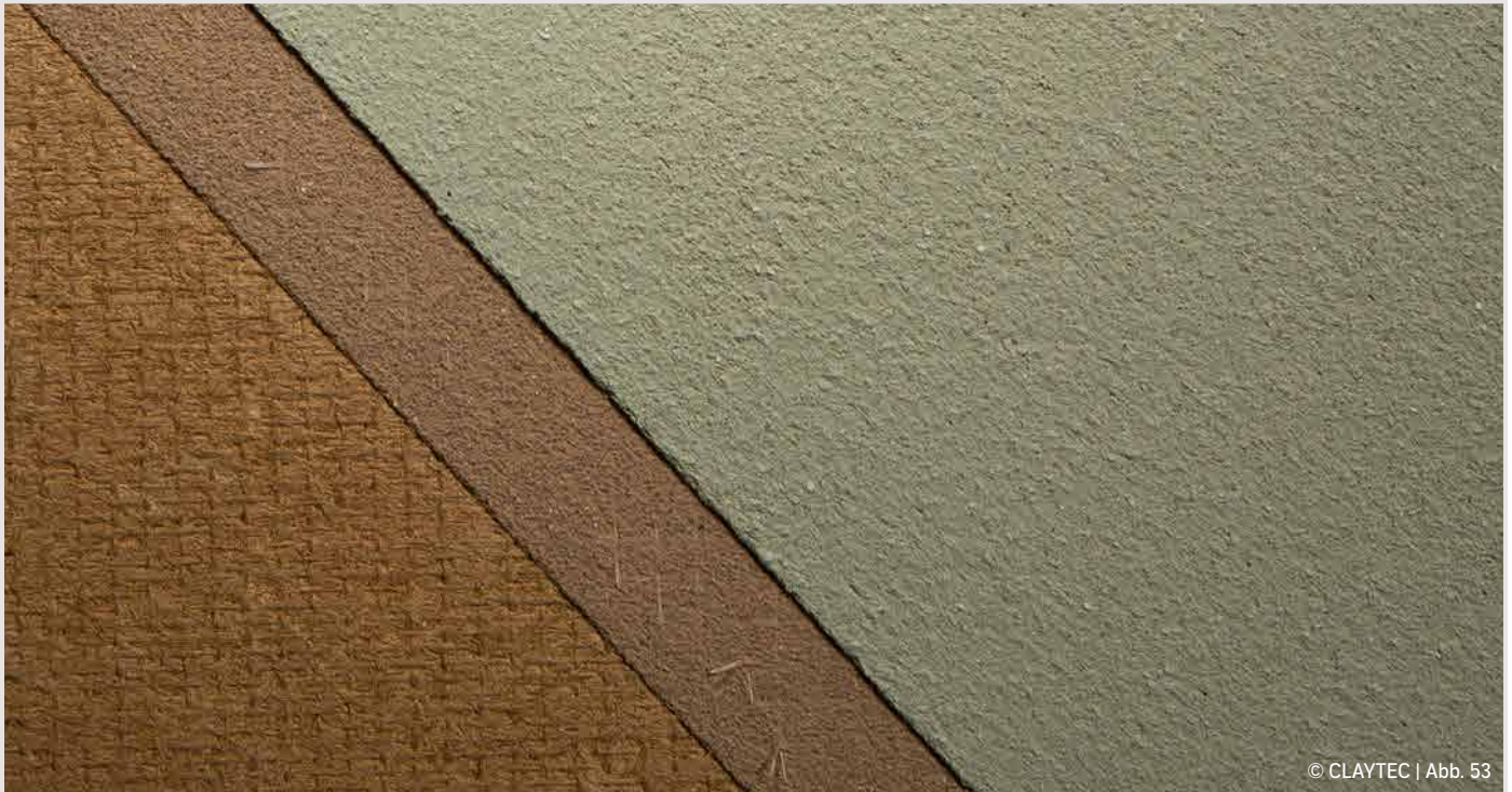
CLAYTEC Lehmbauplatte D20, CLAYTEC Lehmklebe- und Armierungsmörtel (mit Flachsgewebe), YOSIMA Lehm-Designputz
